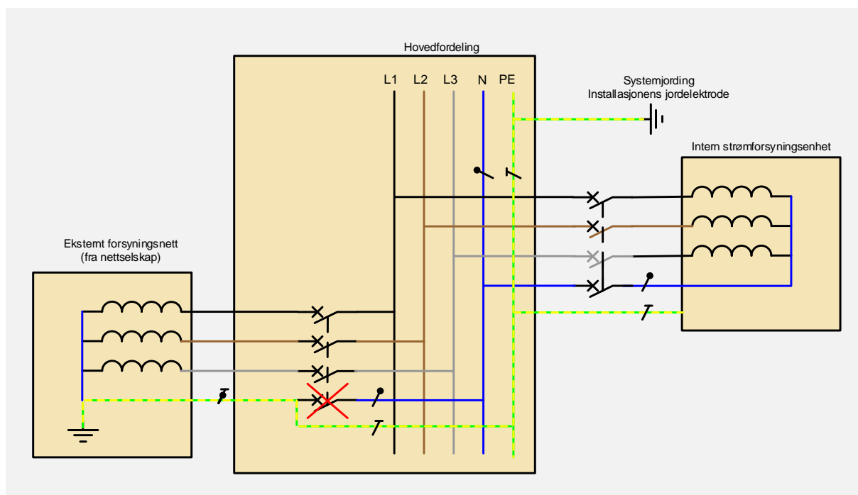
Figur 7: Uakseptabel anvendelse av firepelig vern/bryter i innkommende forsyning fra nettselskap
